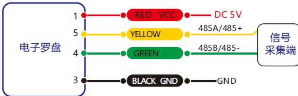
RS 485接线图
