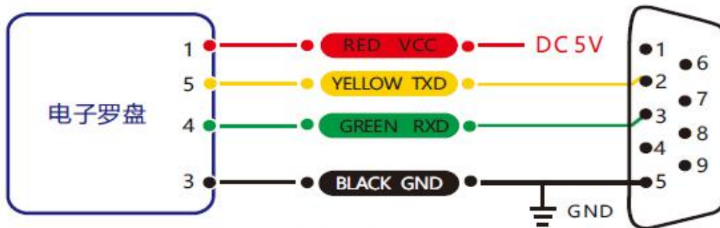
RS 232接线图
